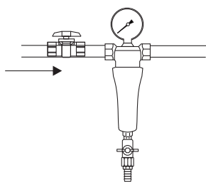
Rys. 2. Montaż narurowy pojedynczego filtra na rurze doprowadzającej gorącą wodę.
