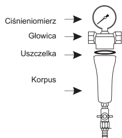
Rys. 1. Części składowe modelu FHMB.
