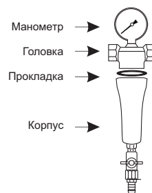
Рис. 1. Составляющие части фильтра FHMB.
